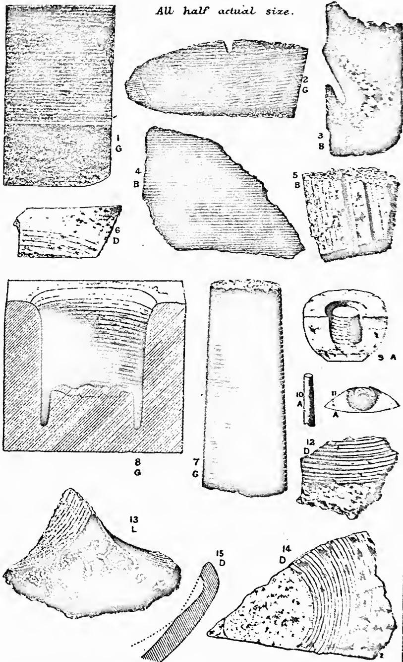
A. Alabaster. B. Basalt D. Diorite. G. Granite. L. Limestone.
